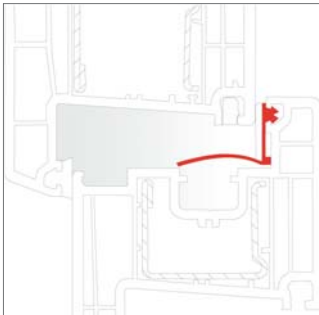
Положение на пластината при стандартен въздушен поток
